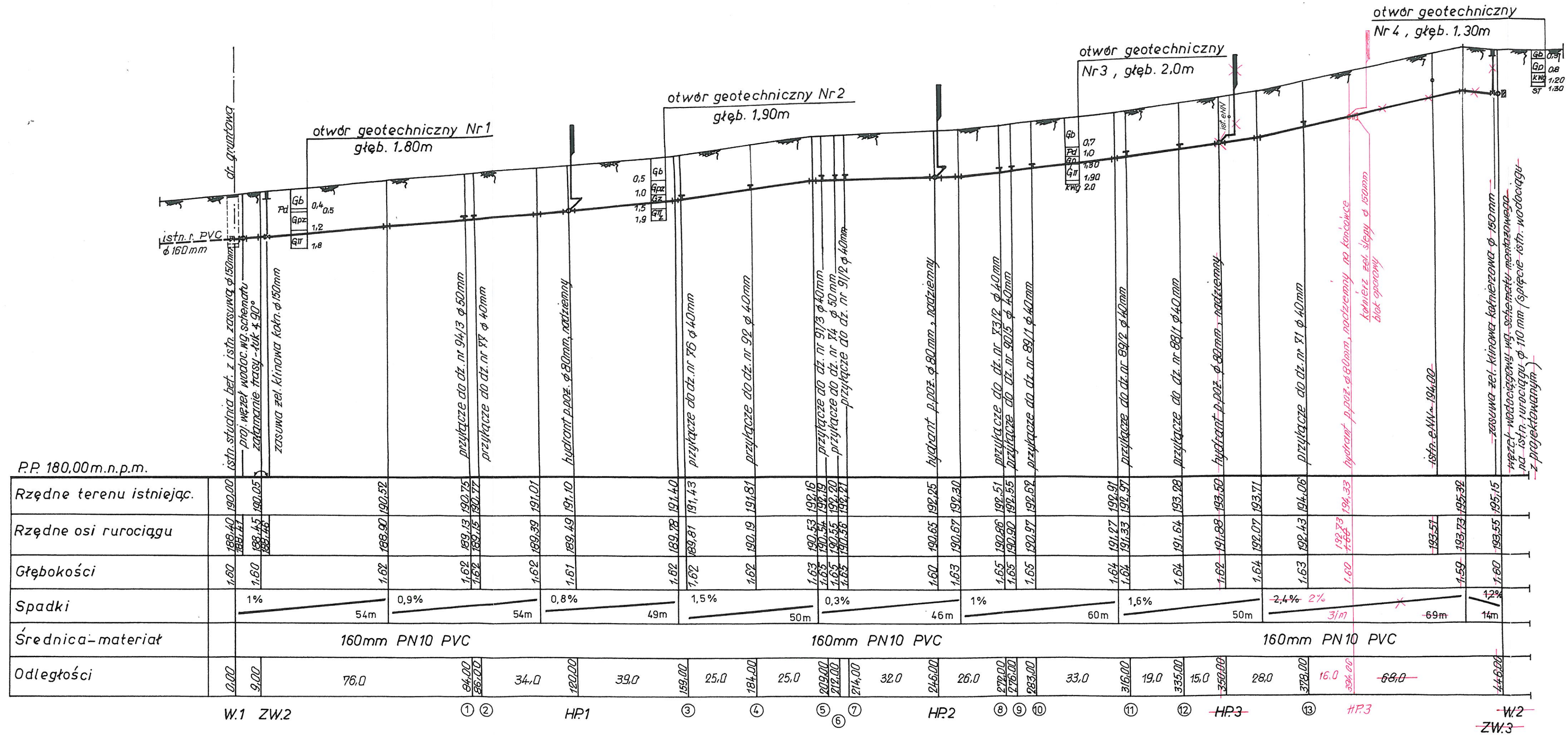
PROFIL PODŁUŻNY SIECI WODOCIĄGOWEJ 1:100/1000
