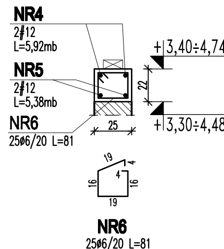
Wieniec W3 2szt. 1:25 L=5.14mb
